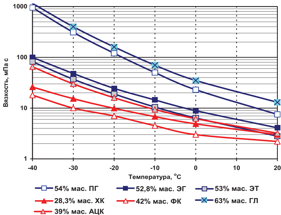
Рисунок 1. Динамическая вязкость хладоносителей с тн.кр. -40°C
