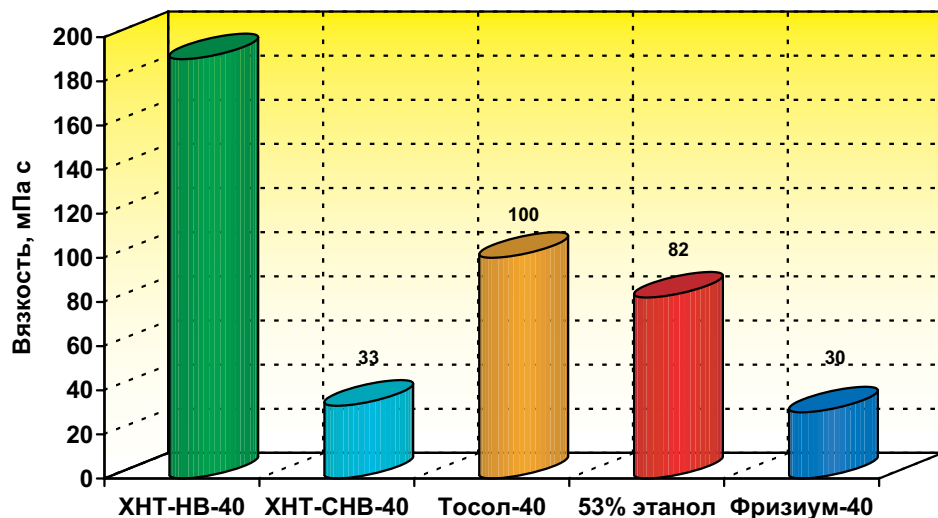
Рисунок 3. Значения вязкости различных хладоносителей с t_{нач. кр.} = -40^{\circ}\text{C} при температуре -40^{\circ}\text{C}
