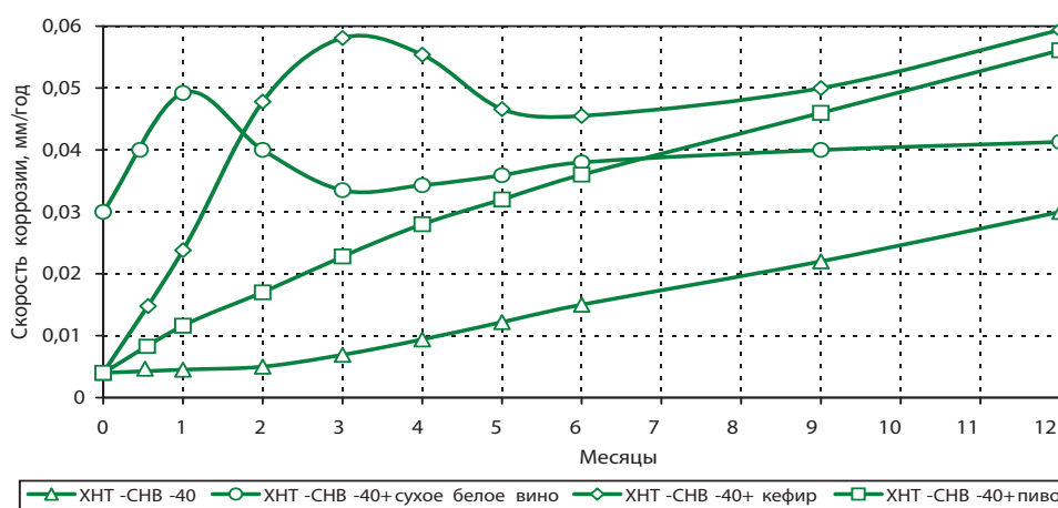
Рисунок 6. Изменение во времени скорости коррозии образца стали Ст20 в хладоносители ХНТ-СНВ-40 при +20°C при протечке в хладоноситель 1% масс. охлаждаемой продукции.
