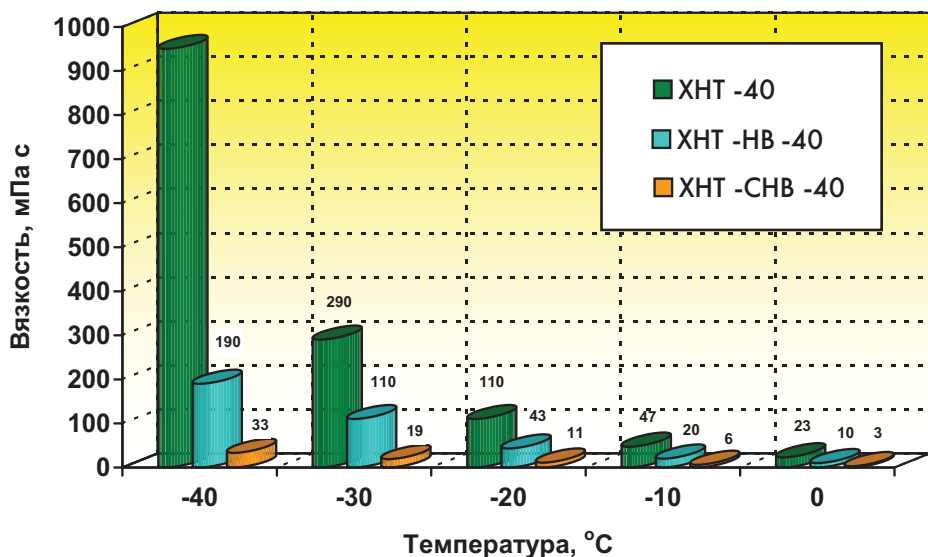
Рисунок 2. Зависимость от температуры вязкости пропиленгликолевых хладоносителей с t_{нач. кр.} = -40^{\circ}\text{C} марок ХНТ, ХНТ-НВ и ХНТ-СНВ.
